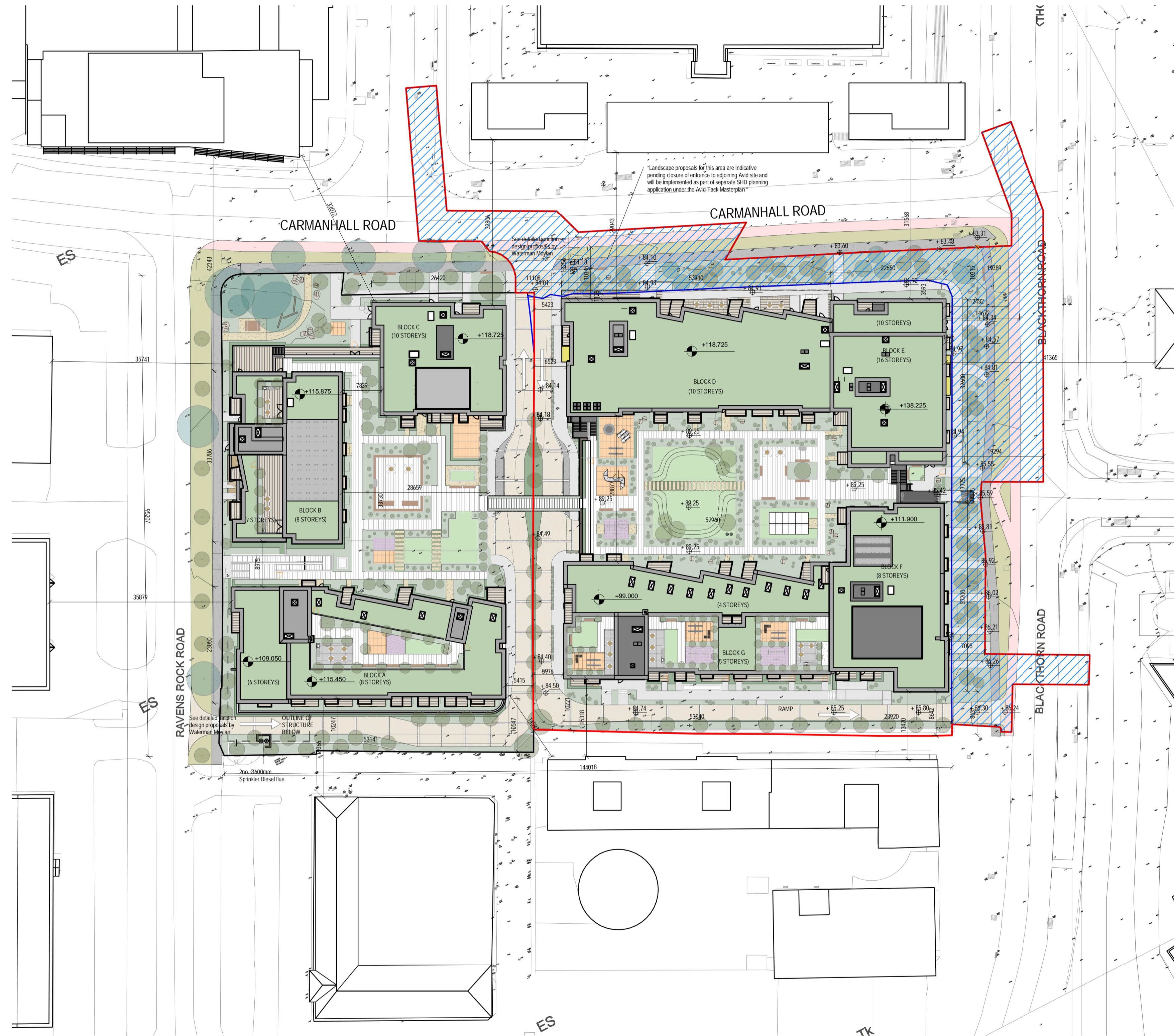
1 SITE PLAN - MASTERPLAN 1 : 500
